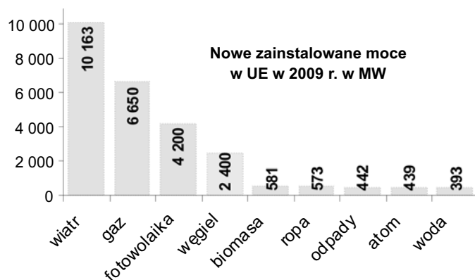
Rys. 2. Nowe moce zainstalowane w Unii Europejskiej w 2009 roku
