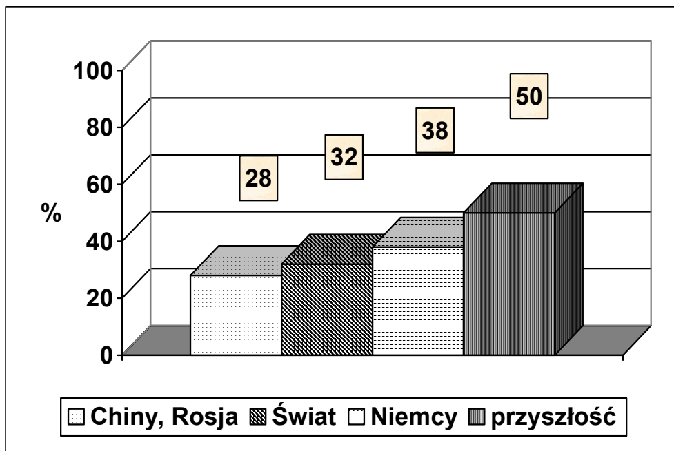
Rys. 3. Sprawność elektrowni na węglu kamiennym w 2000 roku Źródło: (Steinkohle 2000, str. 34).
