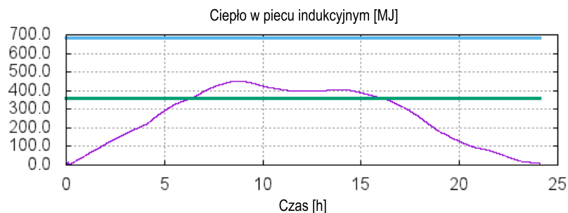
Rys. 3. Ciepło użyteczne w piecu
