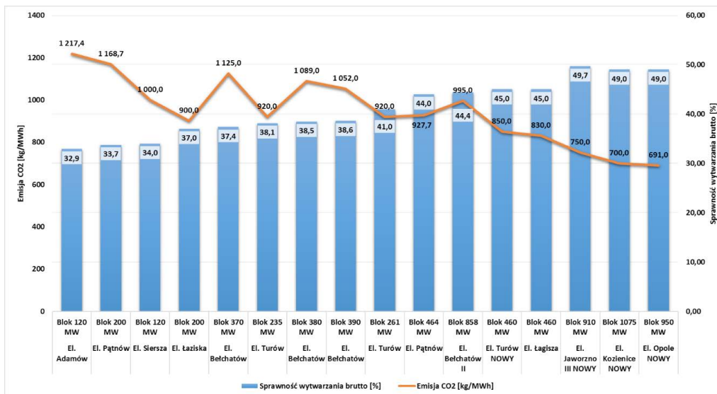
Rys. 8. Porównanie sprawności elektrowni z emisją CO 2 (Kasztelewicz 2014/2015)
