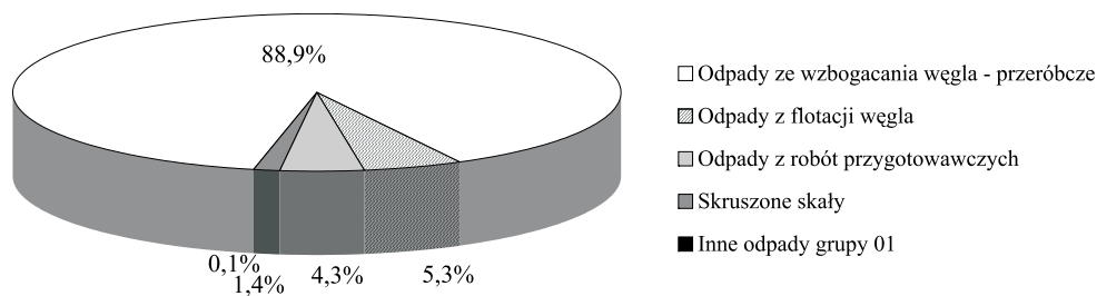
Rys. 2. Struktura rodzajowa wytwarzanych w 2007 r odpadów w kopalniach węgla kamiennego Górnoszląskiego Zagłębia Węglowego [2]
