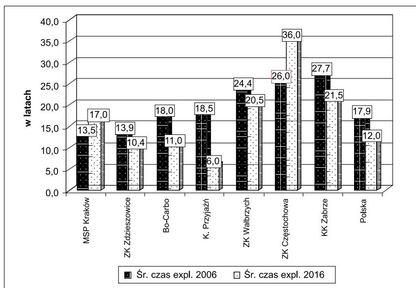
Rys. 1. Zmiana średniego wieku baterii koksowniczych w latach 2006—2016
