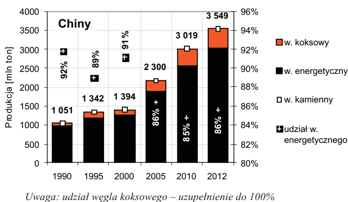
Rys. 2.2. Rozwój produkcji węgla kamiennego w Chinach w latach 1990–2012 Źródło: opracowanie własne na podstawie (Coal Information 2010, 2013)
